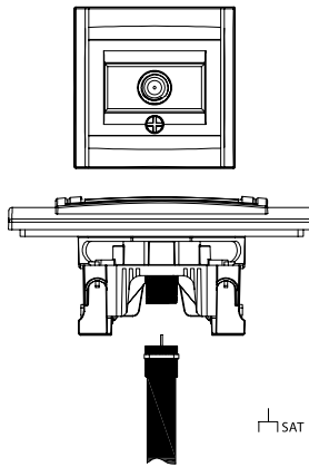
SAT Socket Outlet F Type (Rg6 F Connector) Uydu Prizi (Rg6 F Konnektörlü) XXX-XXXXXX-180
