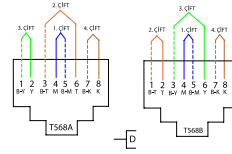
Connection Options TIA - 568 Bağlantı Seçenekleri
