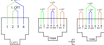
Connection Options TIA - 568 Bağlantı Seçenekleri
