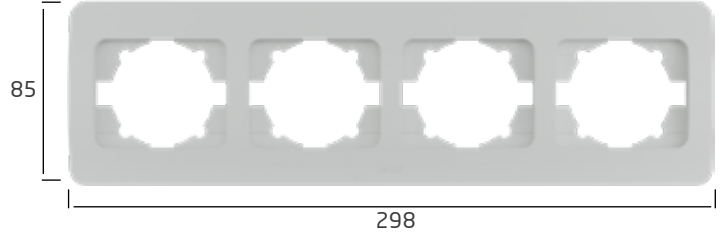
4 Gang Frame / Dörtlü Çerçeve 508-01XX00-228
