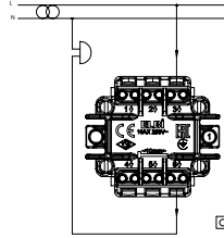
2Gang 2Way Switch Komütatör Veavien XXX-XXXXXX-211
