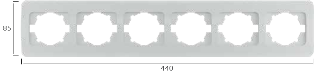
6 Gang Frame / Altılı Çerçeve 508-01XX00-252
