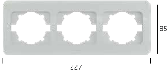
3 Gang Frame / Üçlü Çerçeve 508-01XX00-227
