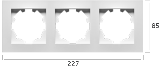
3 Gang Frame / Üçlü Çerçeve 510-01XX00-227
