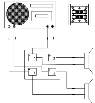
Music Hi-Fi Socket 2 Gang İkili Müzik Yayın Prizi XXX-XXXXXX-241
