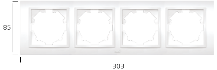
4 Gang Frame / Dörtlü Çerçeve 500-01XX00-228
