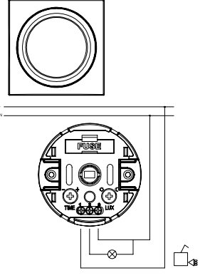
Triac Motion Sensor Triyaklı Hareket Sensörü XXX-XXXXXX-264
