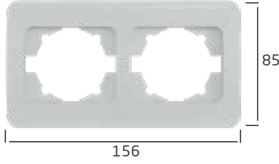
2 Gang Frame / İkili Çerçeve 508-01XX00-226
