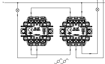
2Gang 1Way Control Switch Light Komütatör Light XXX-XXXXXX-257
