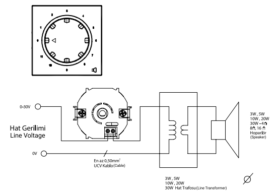
Music Volume Control Switch Müzik Yayın Anahtarı XXX-XXXXXX-261
