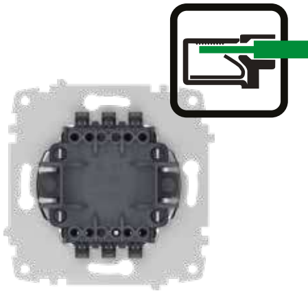
Quick Connect (screwless) Hızlı Bağlantı (vidasız)
