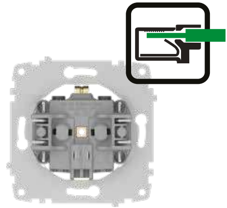
Quick Connect (screwless) Hızlı Bağlantı (vidasız)
